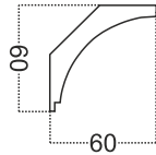
Kr321K (60*60*2000мм)
