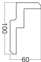
Kr341K (100*60*2000мм)
